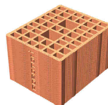
Blocco POROTON® denominato "P700 KLIMA 30x19x25", dimensioni nominali 300 x 250 x 190 mm
