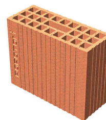
Blocco POROTON® denominato "P800 KLIMA 12x24x30", dimensioni nominali 300 x 120 x 240 mm
