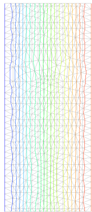
Figura 2 - Mesh dell'elemento ed andamento delle isoterme.
