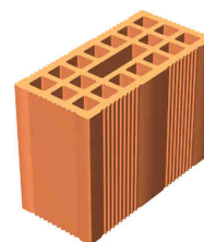
Elemento in laterizio denominato "DOPPIO UNI 12x19x25", dimensioni nominali 250 x 120 x 190 mm
