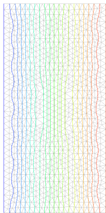
Figura 2 - Mesh dell'elemento ed andamento delle isoterme.
