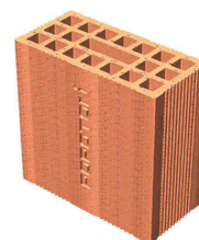
Blocco POROTON® denominato "P800 KLIMA 12x24x25", dimensioni nominali 250 x 120 x 240 mm
