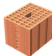
Blocco POROTON® denominato "P800 KLIMA 20x19x25", dimensioni nominali 200 x 250 x 190 mm
