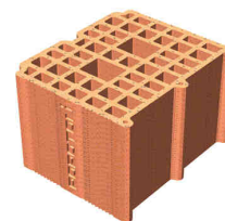
Blocco POROTON® denominato "P800 KLIMA Inc 30", dimensioni nominali 245 x 300 x 190 mm
