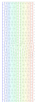
Figura 2 - Mesh dell'elemento ed andamento delle isoterme.
