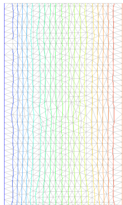
Figura 2 - Mesh dell'elemento ed andamento delle isoterme.
