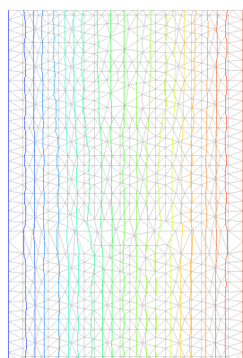
Figura 2 - Mesh dell'elemento ed andamento delle isoterme.
