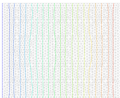
Figura 2 - Mesh dell'elemento ed andamento delle isoterme.
